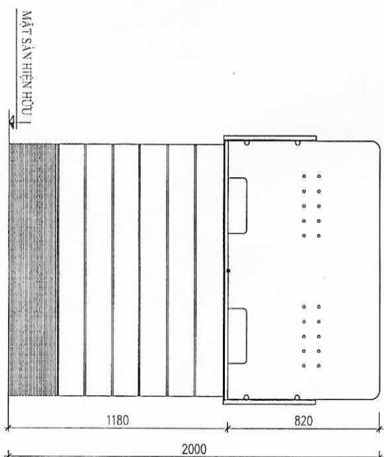
MẶT ĐỪNG BÀN LÀM VIỆC tỷ lệ 1/20
