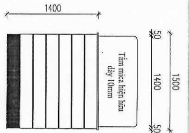
MẶT HÔNG BÚC LÀM VIỆC CẠCK tỷ lệ 1/40
