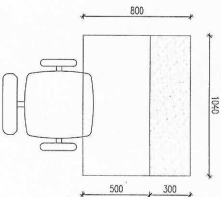
MẶT BẢNG BÀN LÀM VIỆC tỷ lệ 1/20
