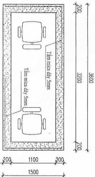
MẶT BÀNNG BÚC LÀM VIỆC CẠCK tỷ lệ 1/40
