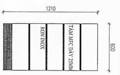
MẶT HÔNG BÀN LÀM VIỆC tỷ lệ 1/20
