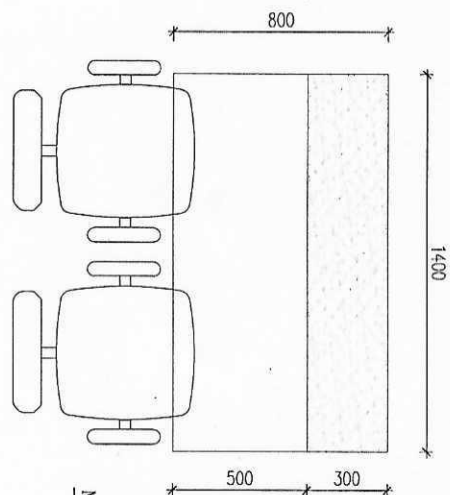
MẶT BẢNG BÀN LÀM VIỆC tỷ lệ 1/20
