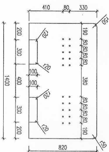
CHI TIẾT TÀM MICA tỷ lệ 1/20
