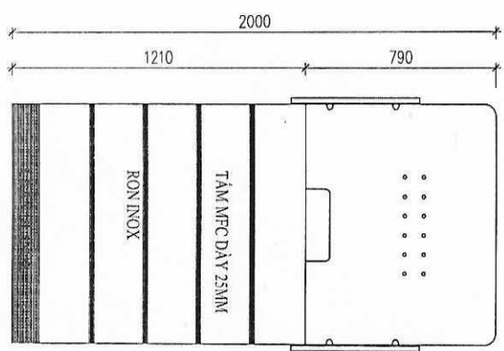
MẶT ĐỪNG BÀN LÀM VIỆC tỷ lệ 1/20
