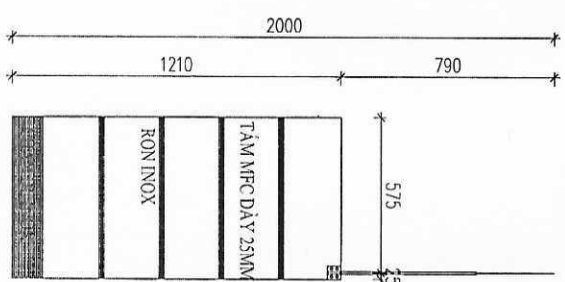
MẶT HÔNG BÀN LÀM VIỆC tỷ lệ 1/20
