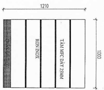
MẶT ĐỪNG BÀN LÀM VIỆC tỷ lệ 1/20
