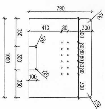
CHI TIẾT TẦM MICA tỷ lệ 1/20
