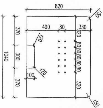
CHI TIẾT TÂM MICA tỷ lệ 1/20
