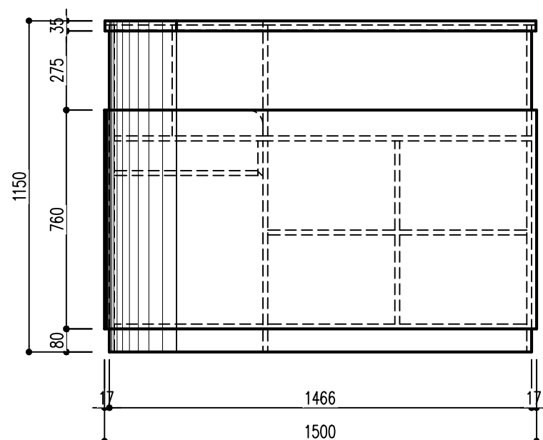
MẶT BÊN NGOÀI QUẦY VÉ
