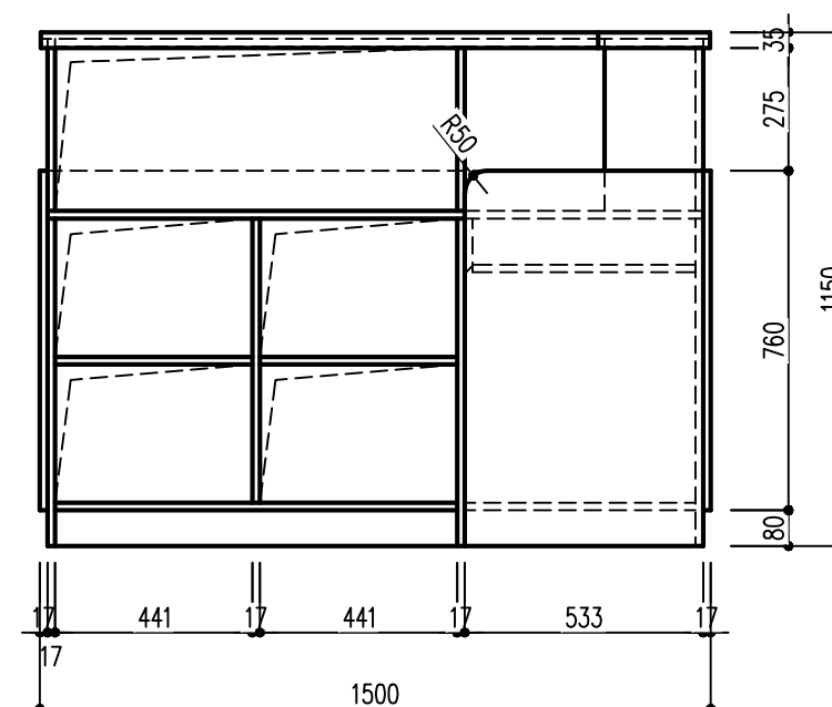
MẶT BÊN TRONG QUẦY VÉ
