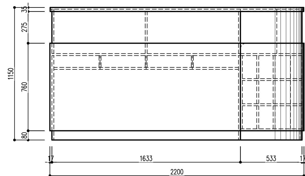
MẶT ĐỨNG NGOÀI QUẦY VÉ
