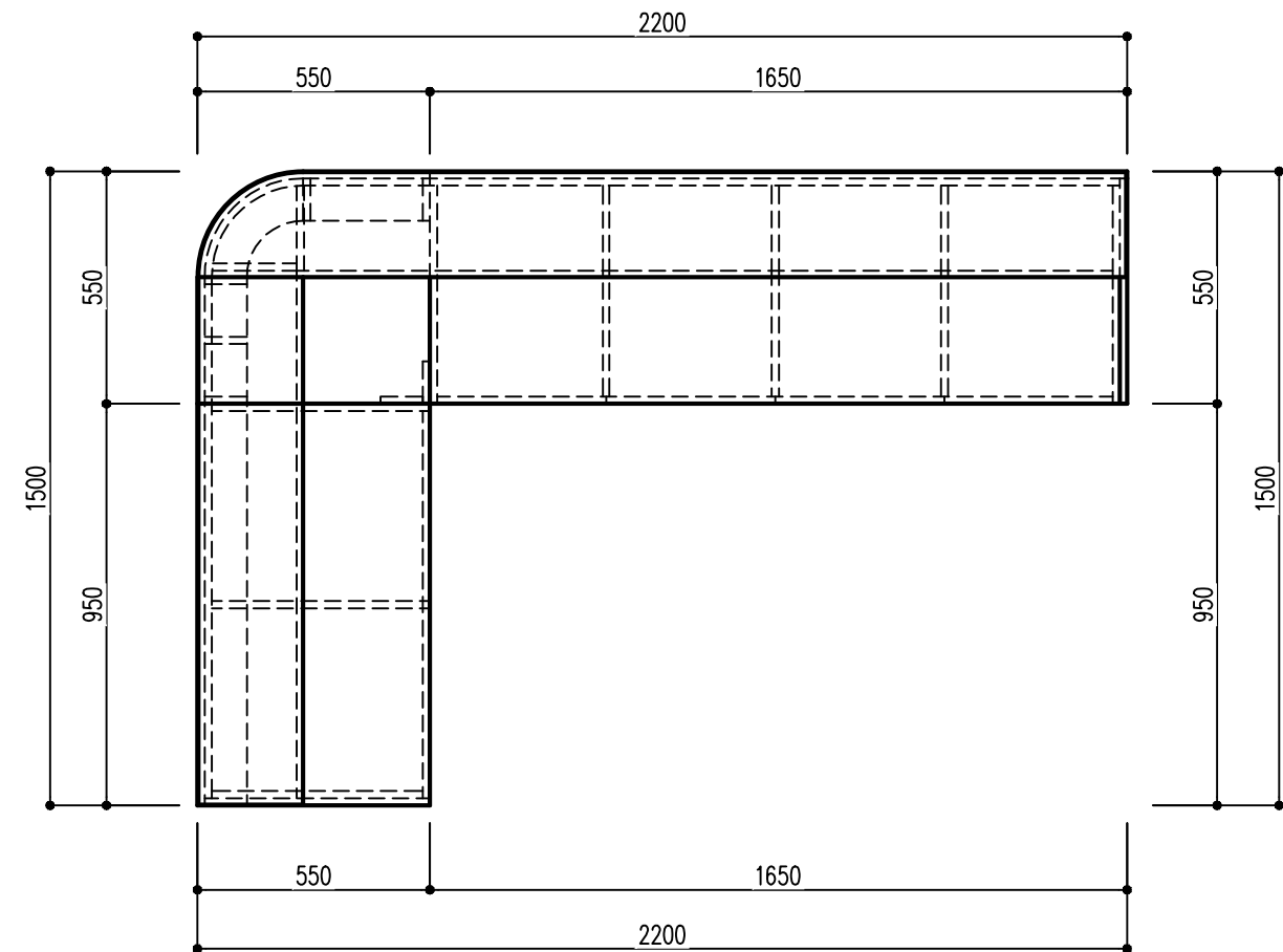
MẶT BẰNG QUẦY VÉ
