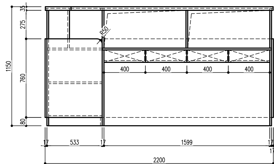
MẶT ĐỨNG TRONG QUẦY VÉ
