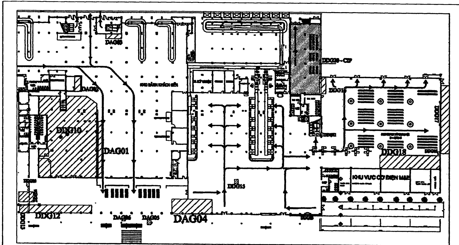
BẢN VẼ MẶT BẰNG PHI HÀNG KHÔNG - TẦNG TRỆT NHÀ GA HÀNH KHÁCH T1 TRẠNG S.21
